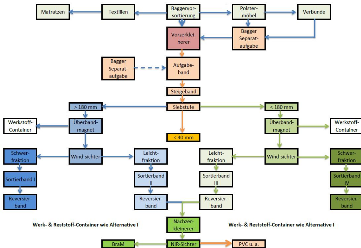
Bild 52: Ausbuanlage – Alternative III (AIII)
