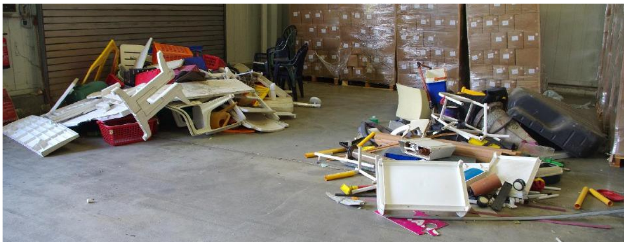
Bild 28: Ergebnis der manuellen Sortierung von Hartkunststoffe aus einer getrennten Sperrmüllsammmlung; links: Gutfraktion; recht: Schlechtfraktion
