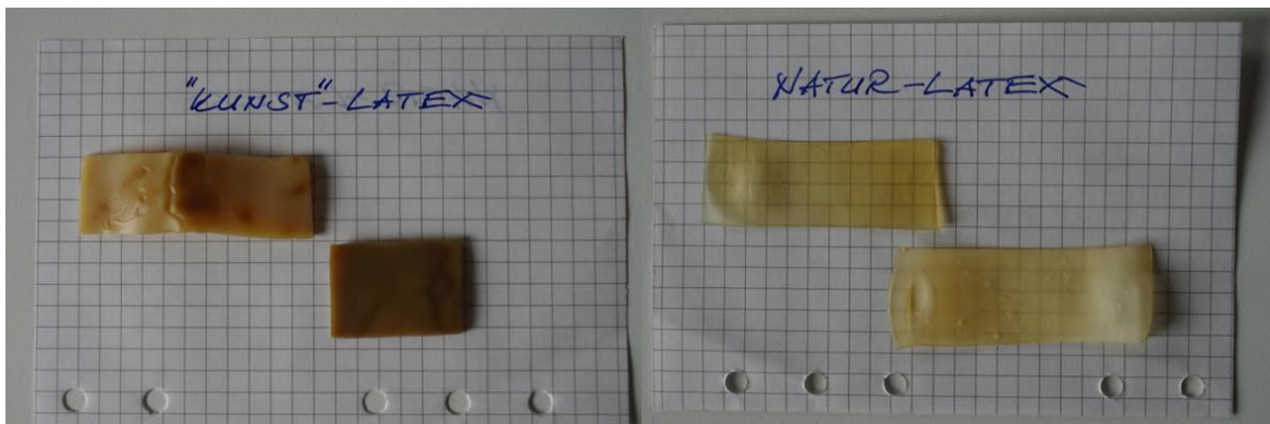
Bild 60: Natur-Latex– „Kunst“-Latex-Proben von einem Matratzenhersteller als Vergleichsprobe
