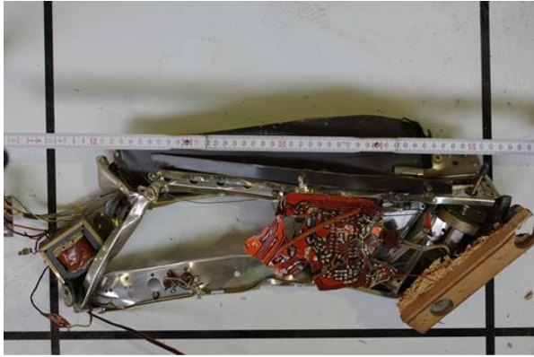
Bild 36: Metallverbund (Elektronik)
