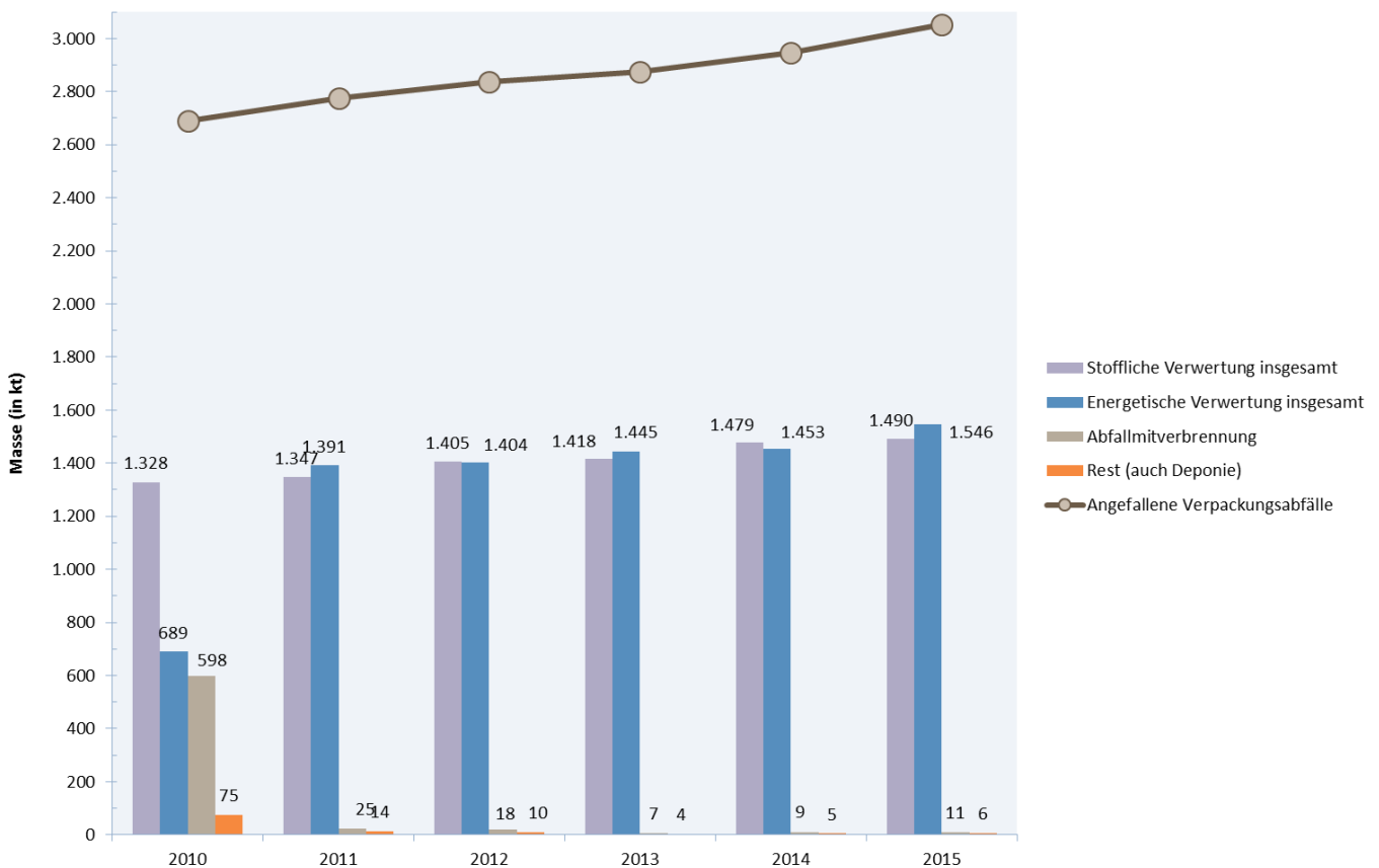
Abbildung 4-3: Entsorgungswege Kunststoffverpackungen (inkl. energetischer Verwertung über den Restmüllpfad)
