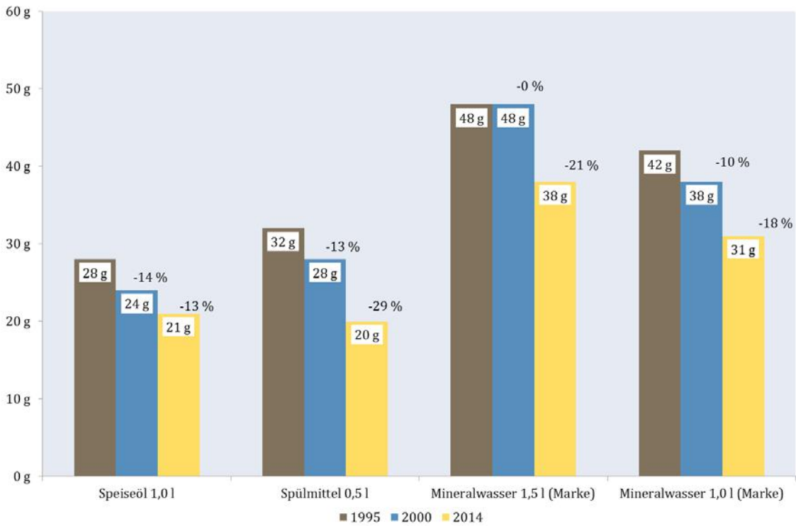
Abbildung 3-40: Entwicklung der Einsatzgewichte von PET-Einwegflaschen für Lebensmittel, Reinigungsmittel und Getränke
