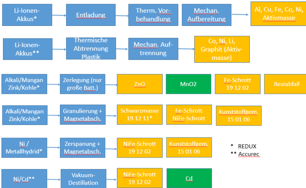
Abb. 5: Recycling von Batterien bei den beiden deutschen Batterieaufbereitern (Quelle: Homepages von REDUX bzw. Accurec und Gespräche mit REDUX); gelb: Zwischenprodukte zur weiteren Verarbeitung, grün: grundsätzlich vermarktbar Endprodukte
