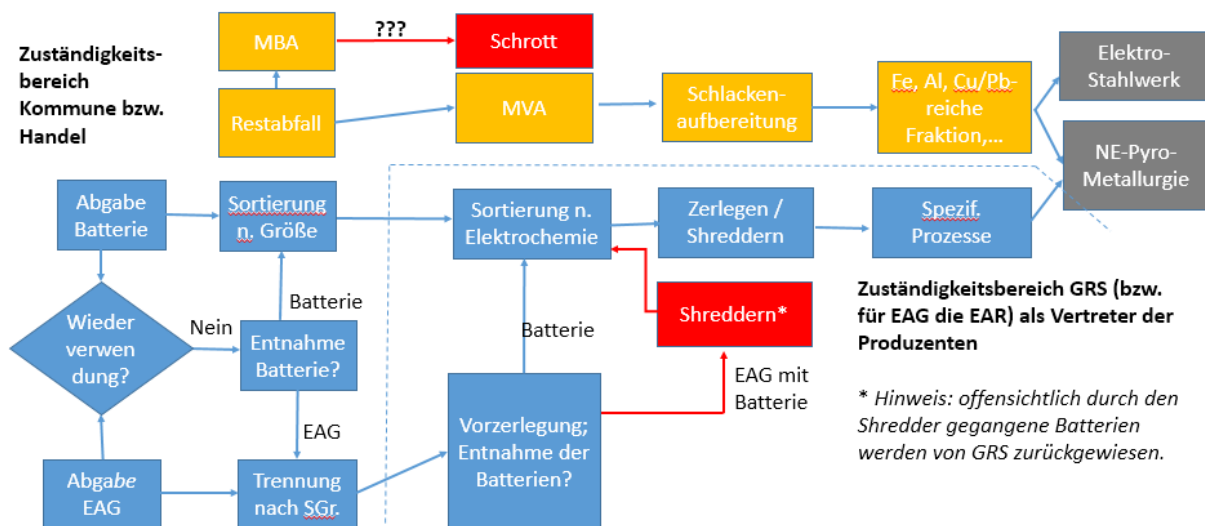
Abb. 2: Stoffstrom Altbatterien (auch aus Elektroaltgeräten); die blauen Kästchen zeigen den Weg der Altbatterien nach getrennter Sammlung, die gelben Kästchen den Weg mit dem Restabfall, die roten Kästchen gefährliche Wege
