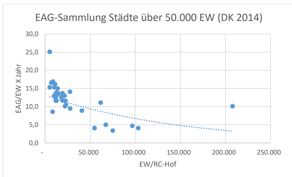
Abb. 4: Sammelmenge an Elektro- und Elektronikaltgeräten in Dänemark als Funktion der Dichte der Wertstoffhöfe
