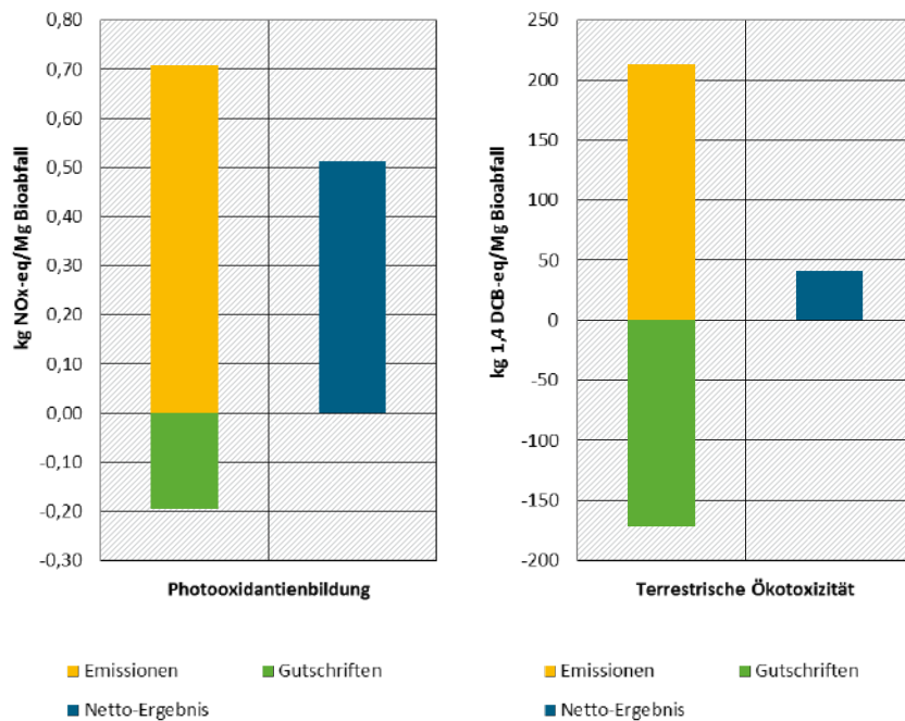
Abbildung 52: Ökobilanzergebnisse (Wirkungskategorien Photooxidantienbildung, terrestrische Ökotoxizität) für das Soldatenfliegenverfahren
