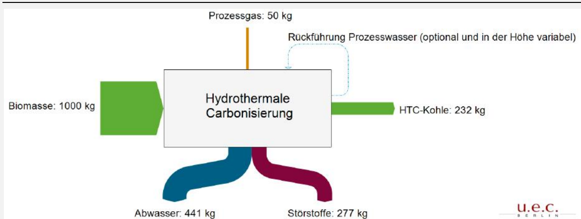
Abbildung 6: Vereinfachte Massenbilanz einer HTC-Anlage bei dem Einsatz von Biomasse (Wassergehalt der Biomasse 40 Ma.-%)
