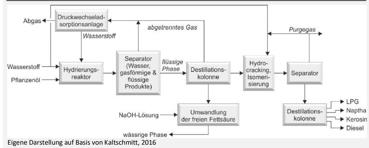
Abbildung 17: Vereinfachtes Prozessschema des HEFA-Verfahrens
