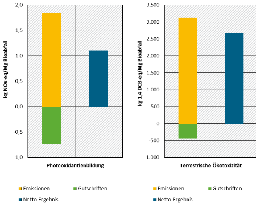
Abbildung 49: Ökobilanzergebnisse (Wirkungskategorien Photooxidantienbildung, terrestrische Ökotoxizität) für die ABE-Fermentation
