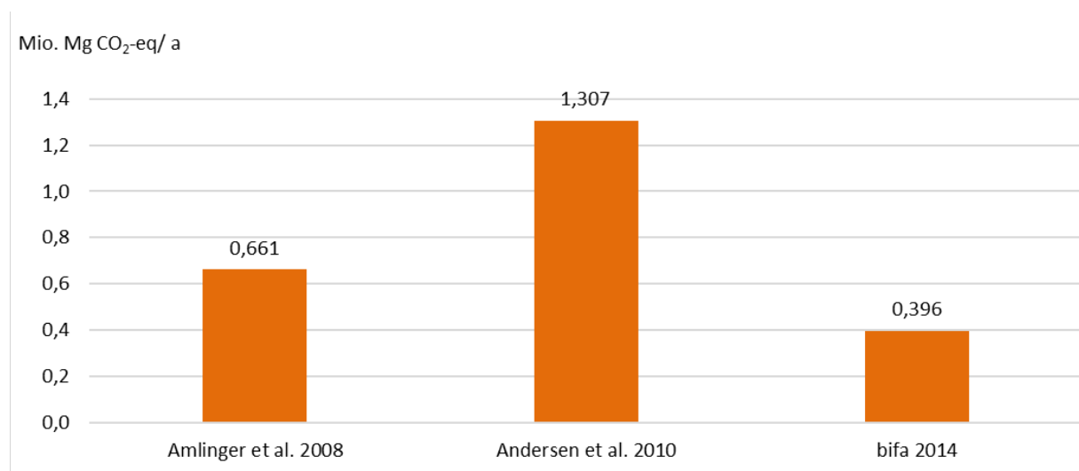
Abbildung 63: Hochrechnung der Emissionen aus der Eigenkompostierung in Deutschland in Mio. Mg CO 2 -eq. pro Jahr
