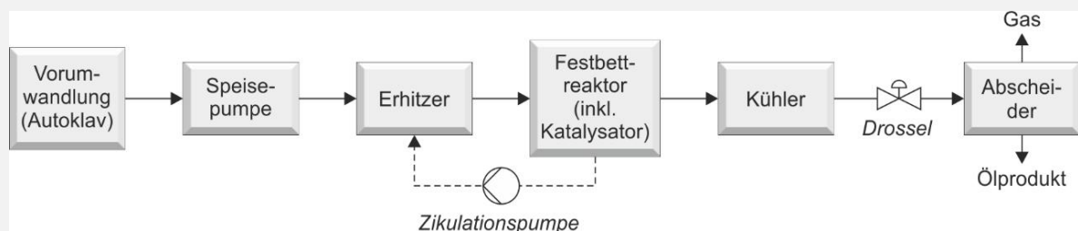
Abbildung 11: Vereinfachtes Prozessschema der kontinuierlichen HTV-Anlage von Licella
