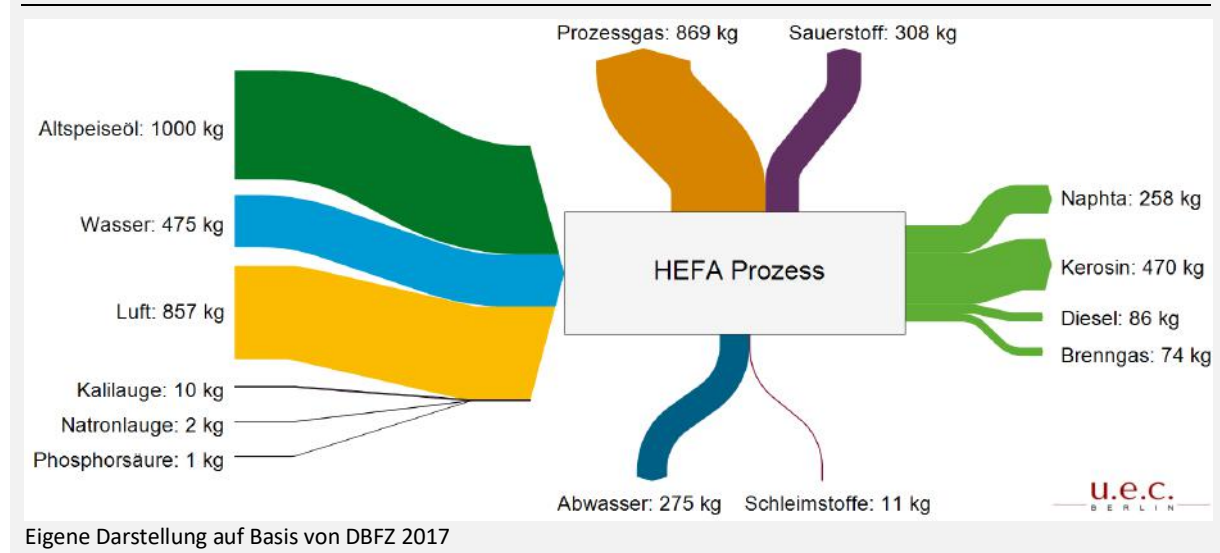
Abbildung 18: Vereinfachte Massenbilanz einer HEFA-Anlage
