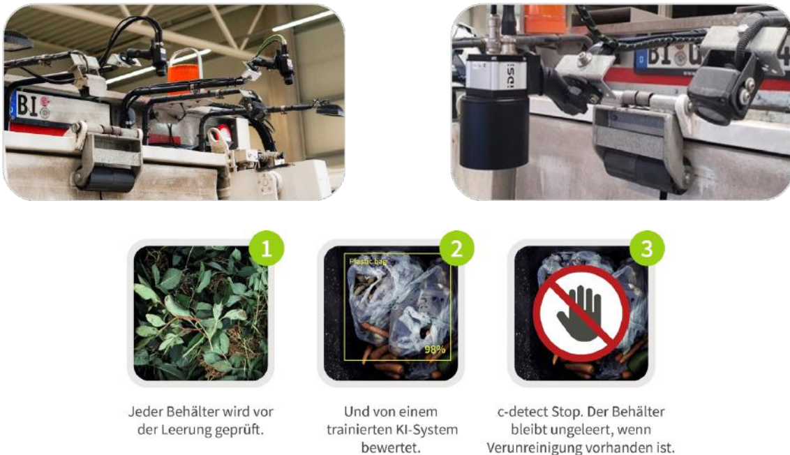
Abbildung 3: Selbsterlernendes Fremdstofferkennungssystem c-detect TopView
