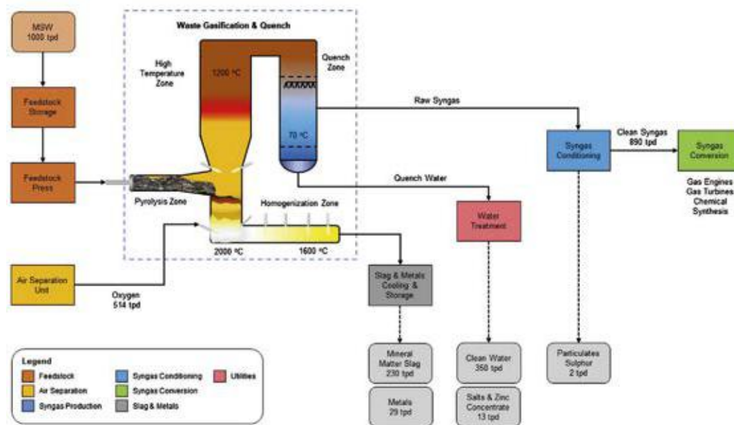
Abbildung 8: Schematische Darstellung des Thermostelect-Verfahrens (Perkins 2020)
