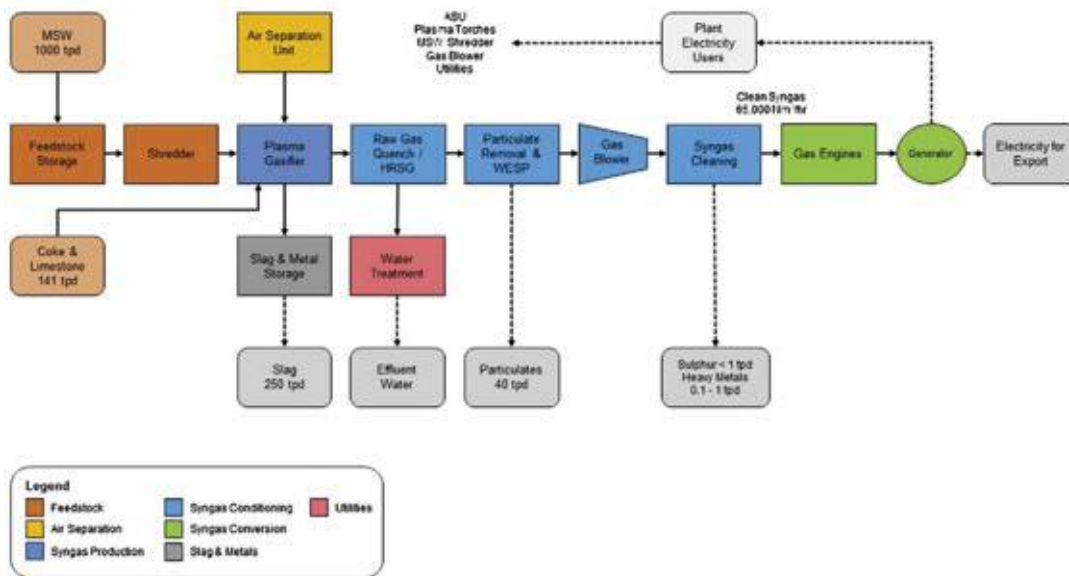
Abbildung 11: Schematische Darstellung des AlterNRG-Verfahrens (Perkins 2020)
