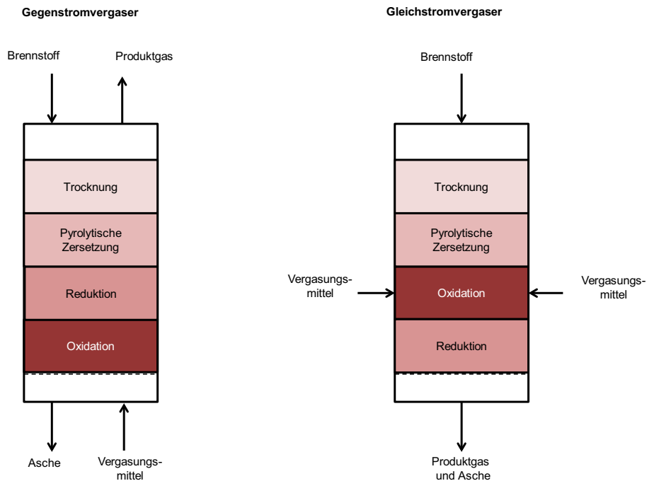
Abbildung 4: Festbettvergaserarten (eigene Darstellung nach Kaltschmitt 2009)
